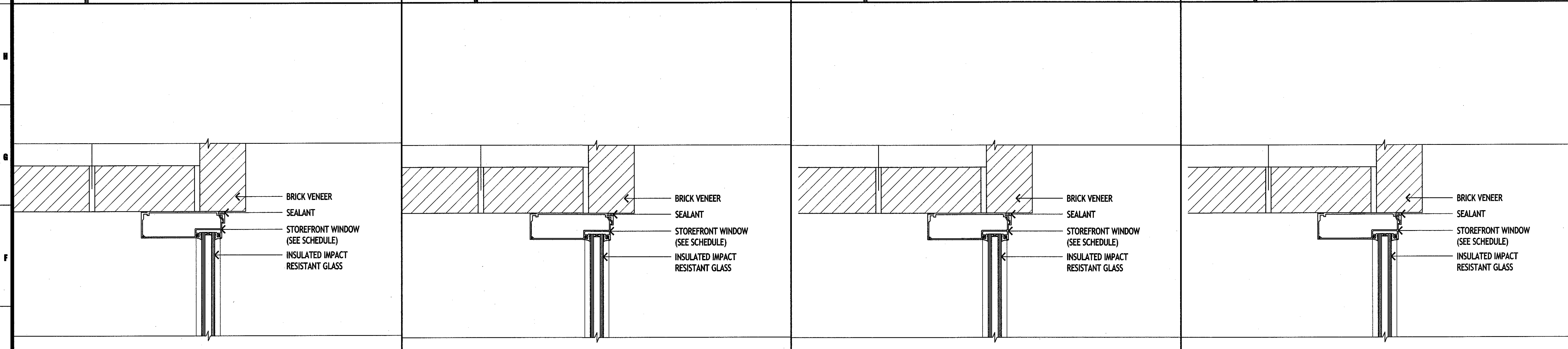
E-1 EXT. STOREFRONT WINDOW JAMB E-5 EXT. STOREFRONT WINDOW JAMB E-9 EXT. STOREFRONT WINDOW JAMB E-13 EXT. STOREFRONT WINDOW JAMB 3\"=1'-0" 3\"=1'-0" 3\"=1'-0" 3\"=1'-0"
