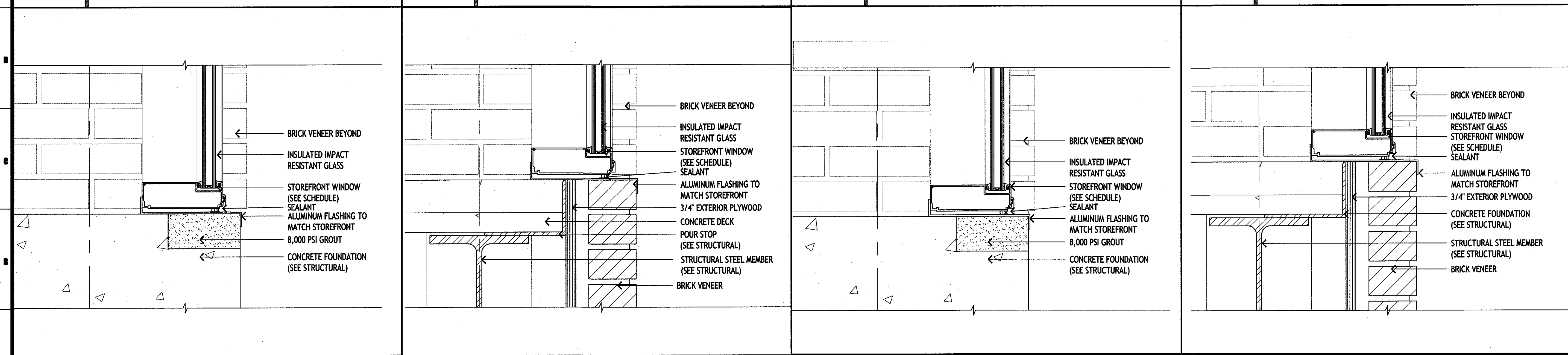
A-1 EXT. STOREFRONT WINDOW SILL A-5 EXT. STOREFRONT WINDOW SILL A-9 EXT. STOREFRONT WINDOW SILL A-13 EXT. STOREFRONT WINDOW SILL 3\"=1'-0" 3\"=1'-0" 3\"=1'-0" 3\"=1'-0"
