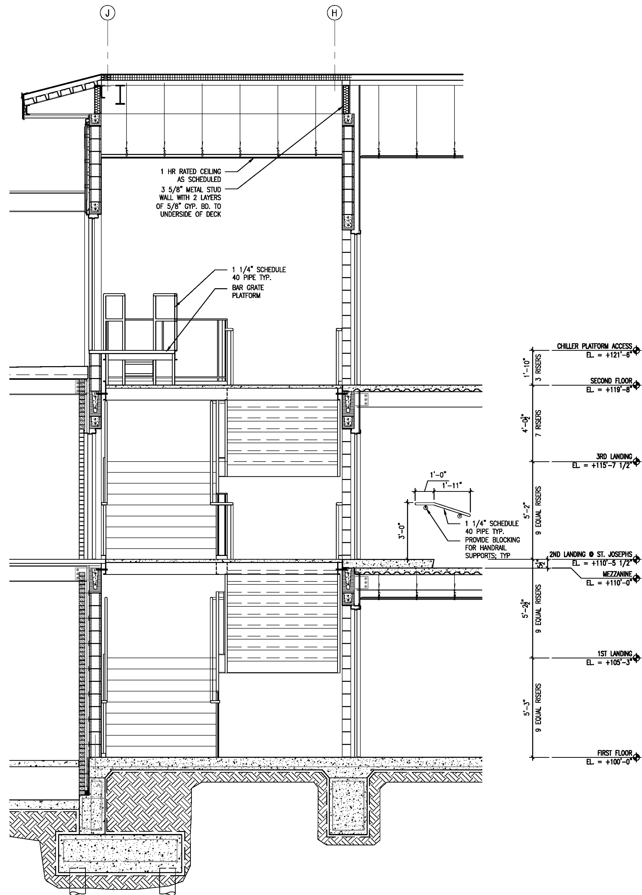
2 SECTION - STAIR B A703 | A704 LOOKING NORTH Scale: 3/8" = 1'-0"
