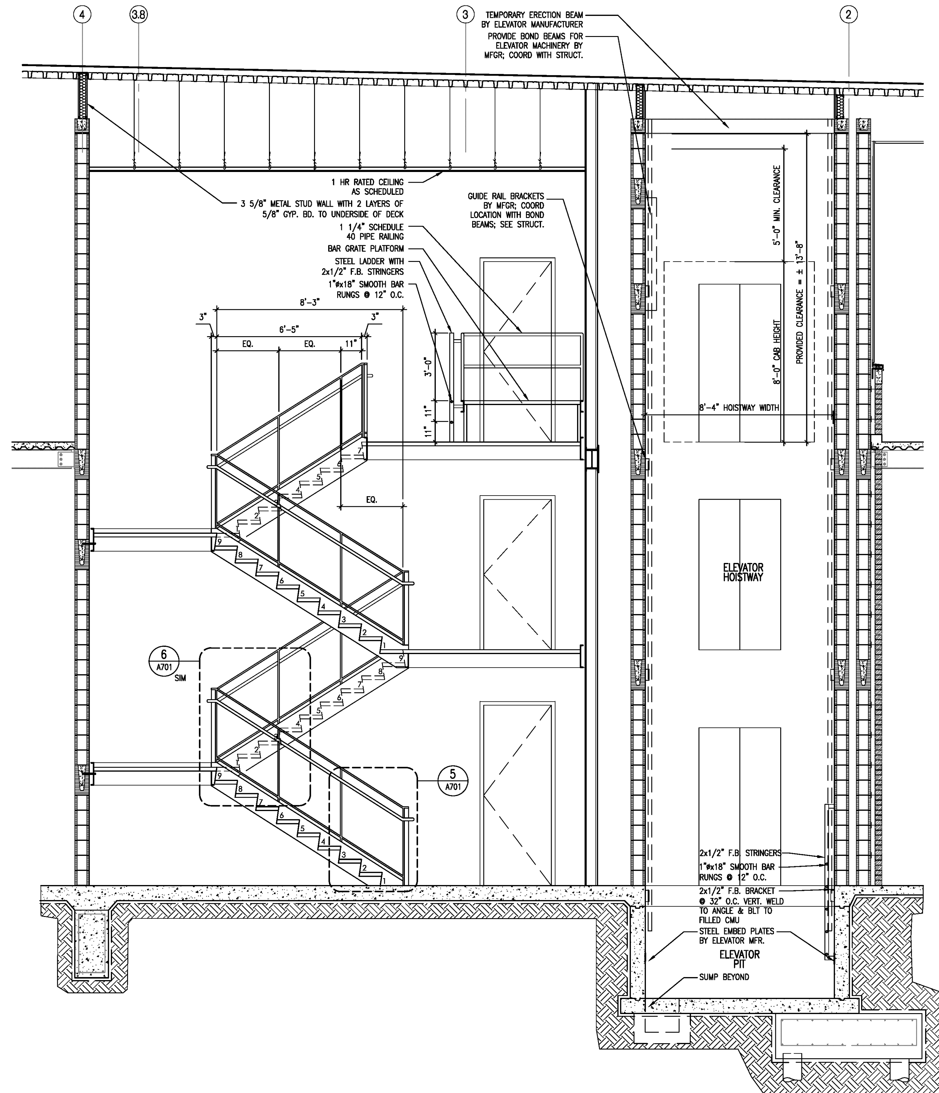
1 SECTION - STAIR B A703 | A704 LOOKING EAST Scale: 3/8" = 1'-0"
