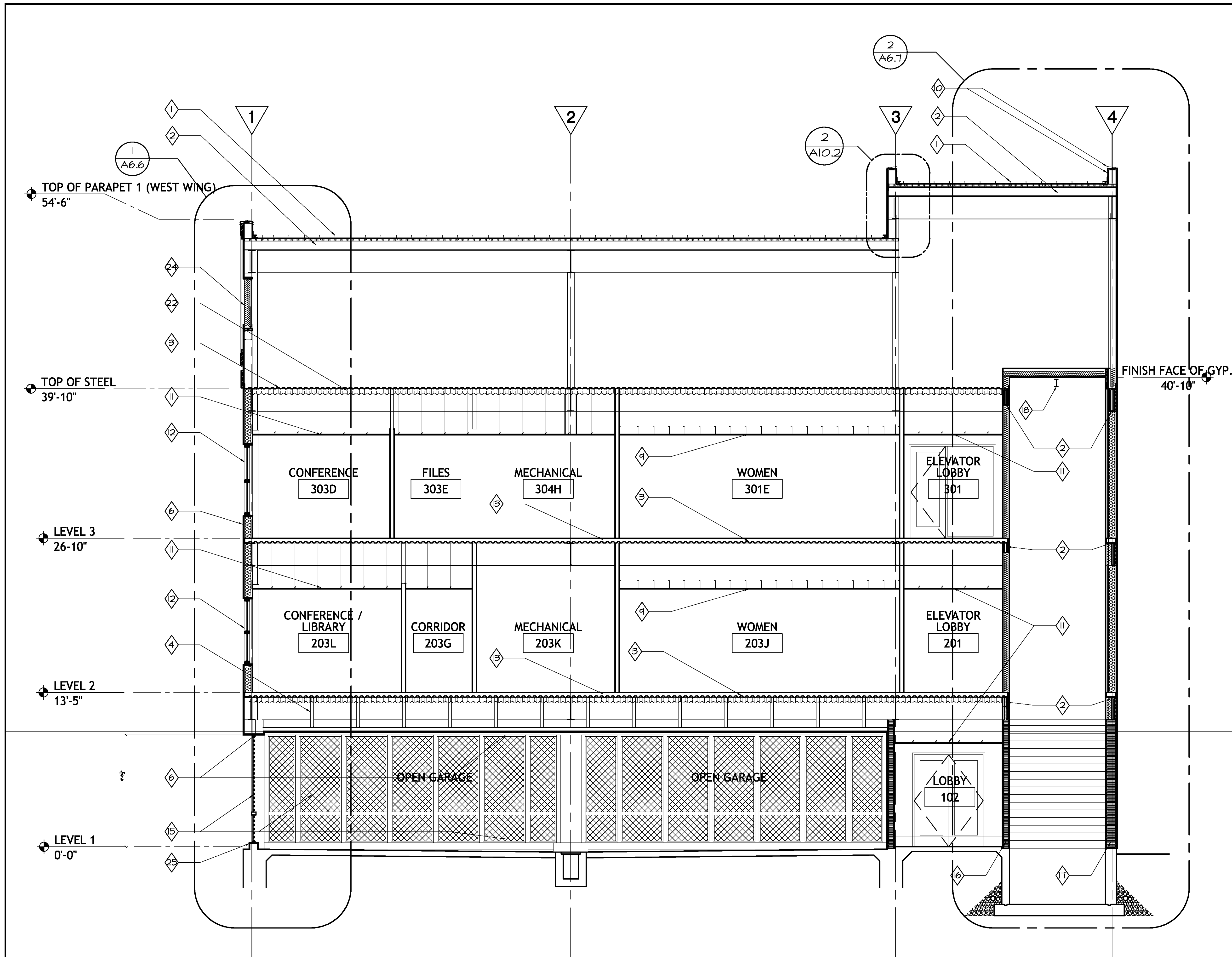
1. BUILDING SECTION - LONGITUDINAL SCALE: 1/4" = 1'-0"
